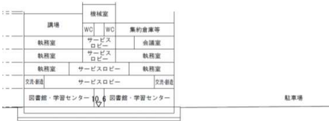
B-B'断面図
