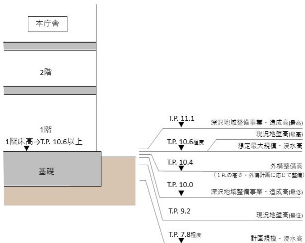
図表 4-4 想定浸水高以上を1FLとする対策イメージ
