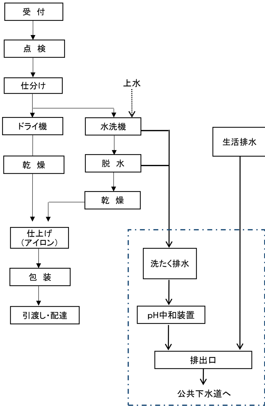
図6 操業の系統と汚水処理の系統
