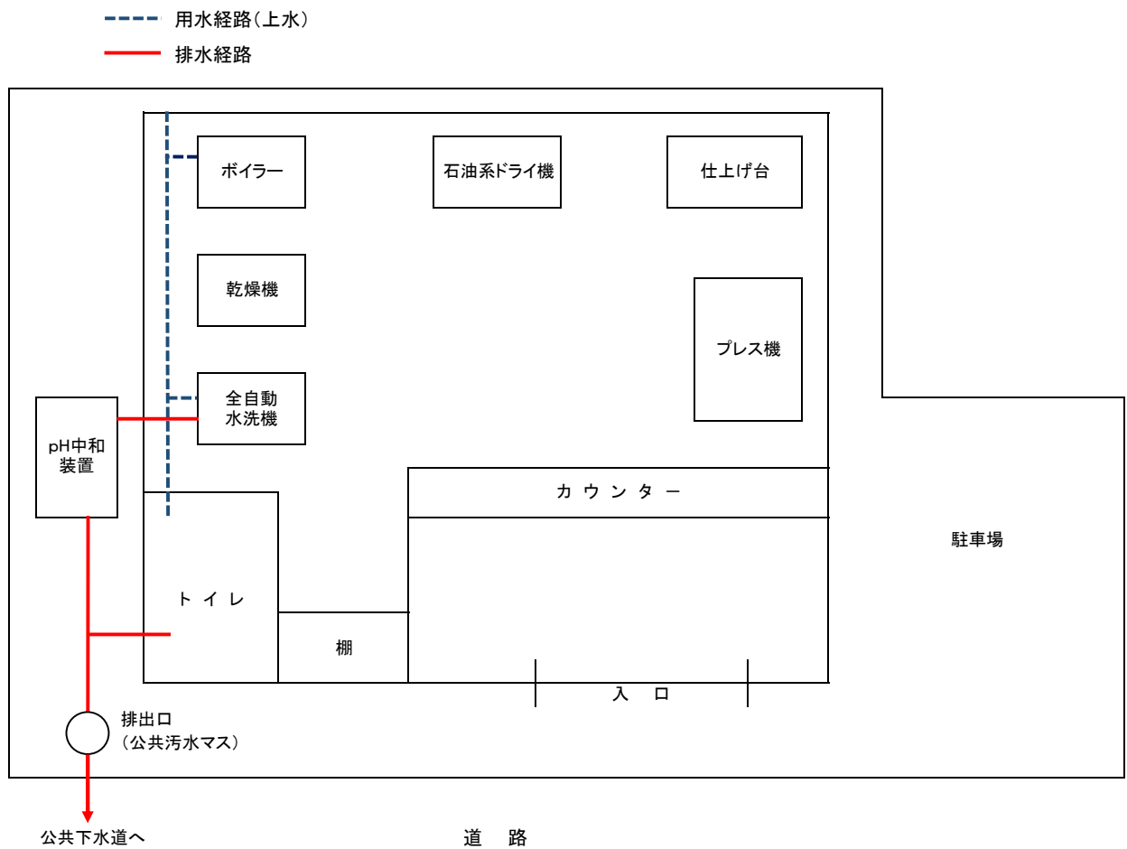
図3 用水及び排水の系統
