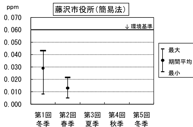
図-2 二酸化窒素の調査結果
