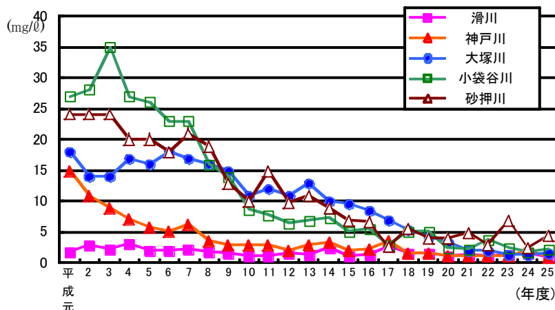
■ 河川水質調査結果(BOD)の推移
