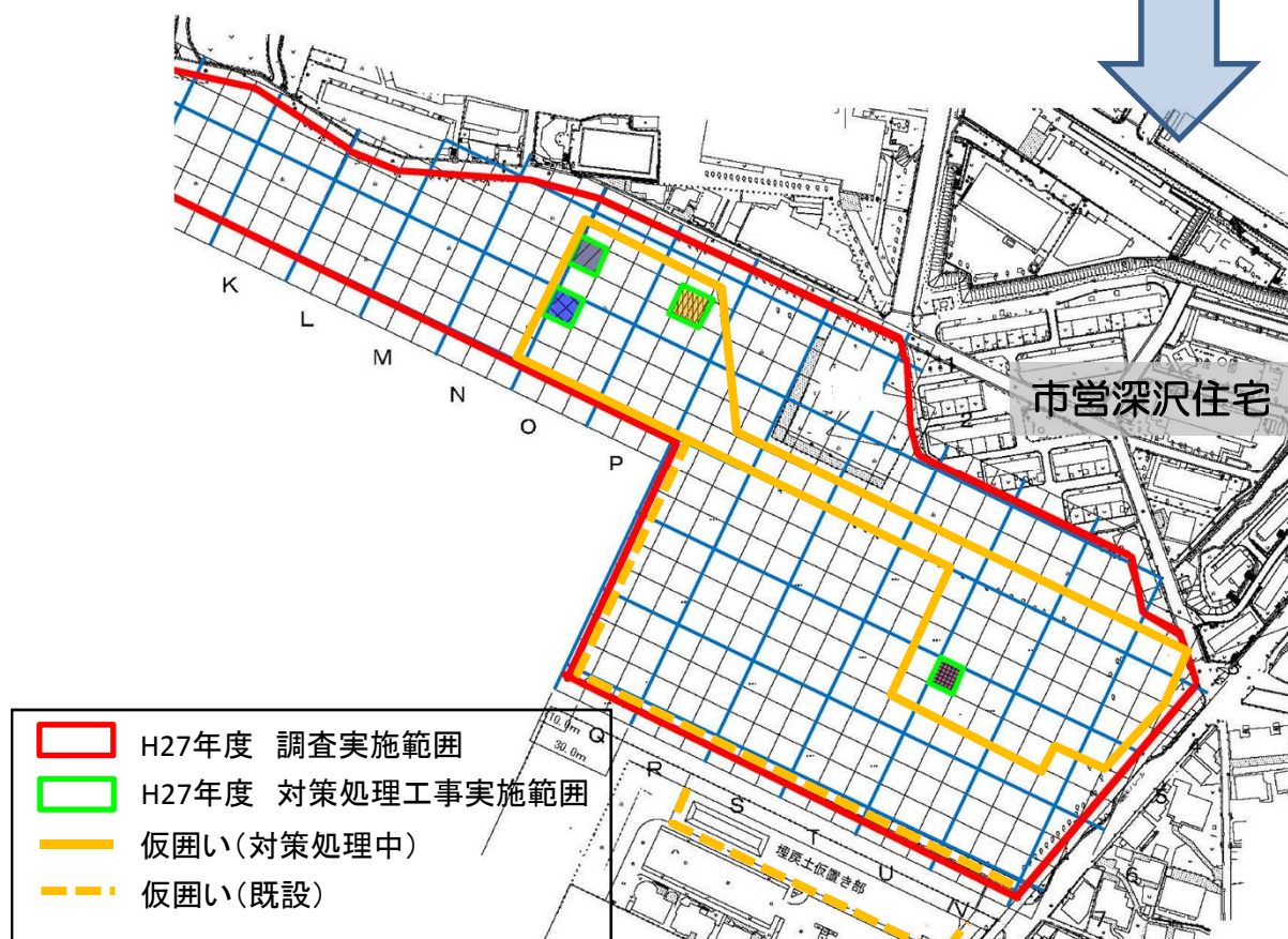
A用地対策工事 実施範囲図
