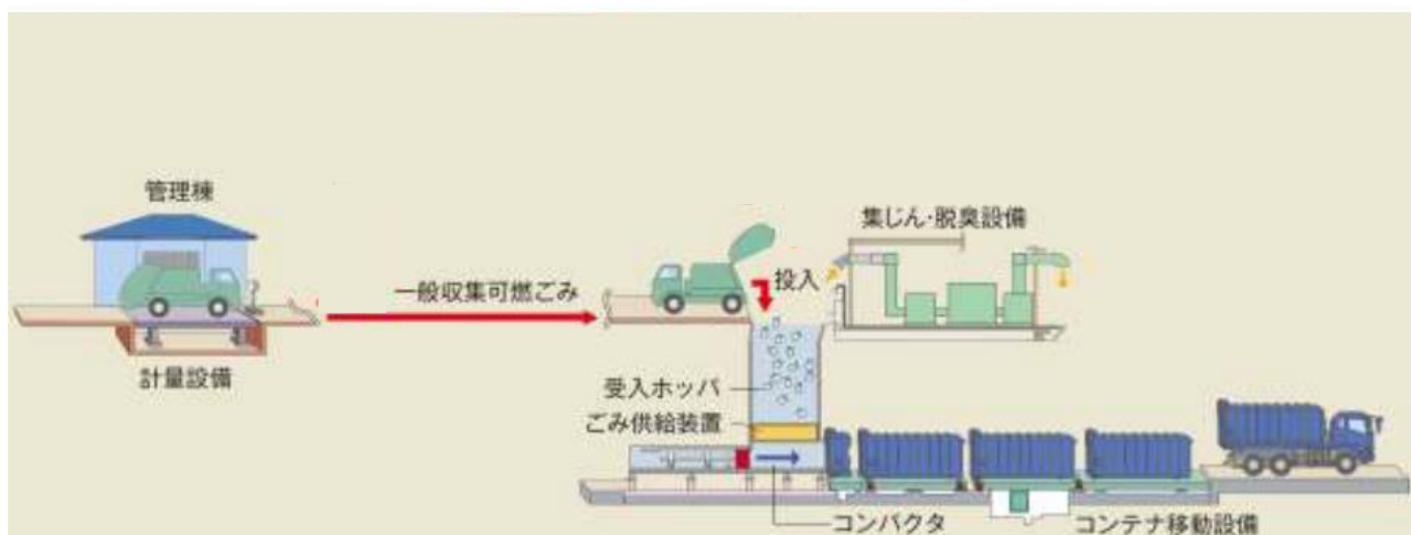
図 4-1 処理フロー
