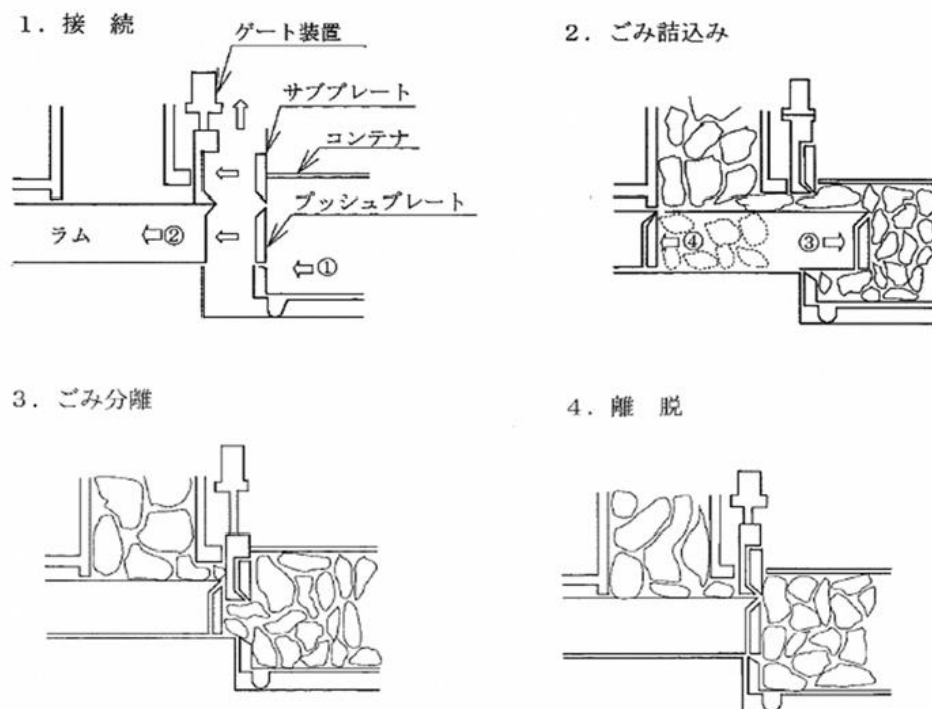
図 5-5 コンパクタ・コンテナ方式の詰込みフロー例
