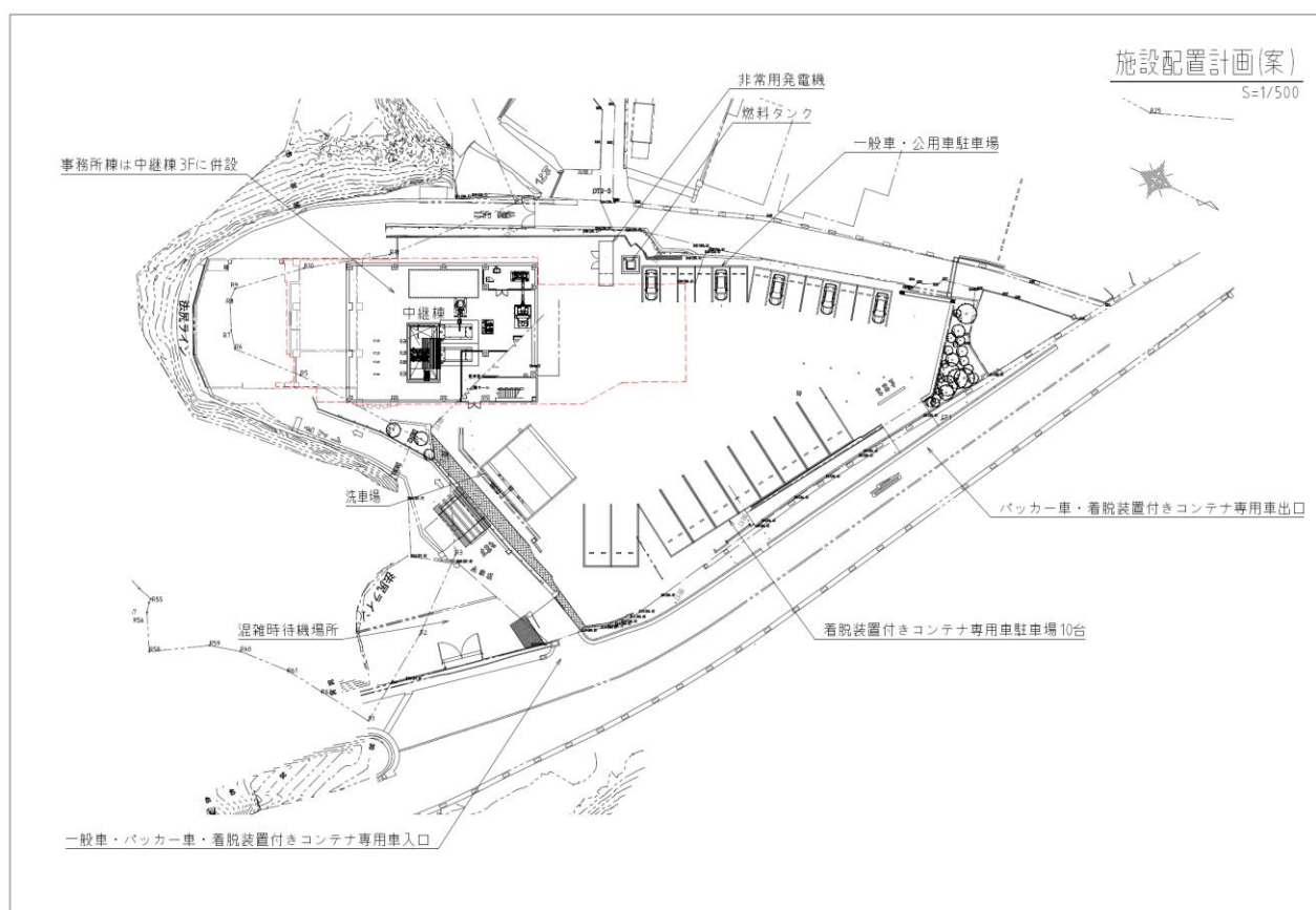
図 5-6 施設配置計画図案
