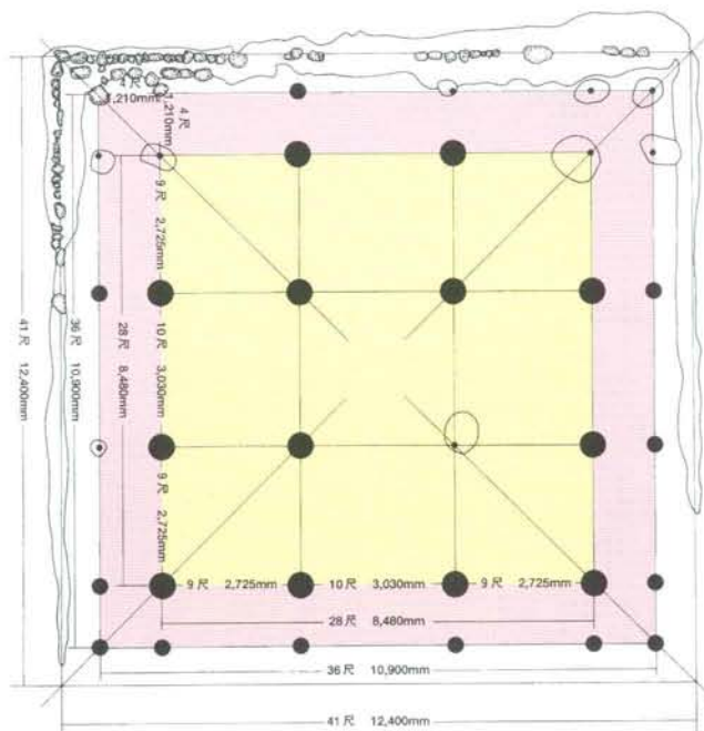
法華堂概念図 Hokedo building shape
